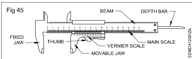
Vernier caliper (Fig 45)
