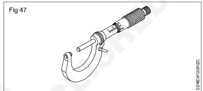
Micrometer (Fig 47)
